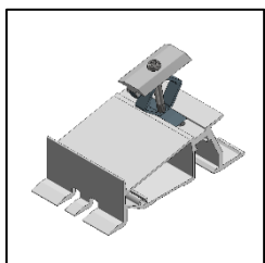
Vorderfuß Mitte 724660
