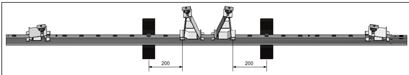
Seitenansicht: 2300mm Abstand
