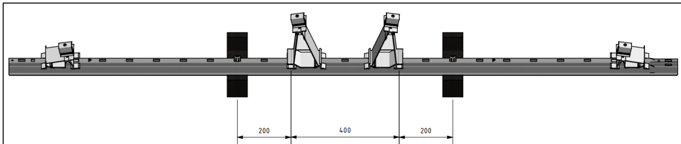
Seitenansicht: 2400mm Abstand
